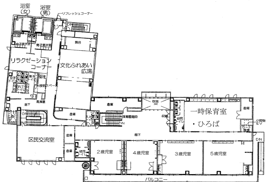
2 階平面図
